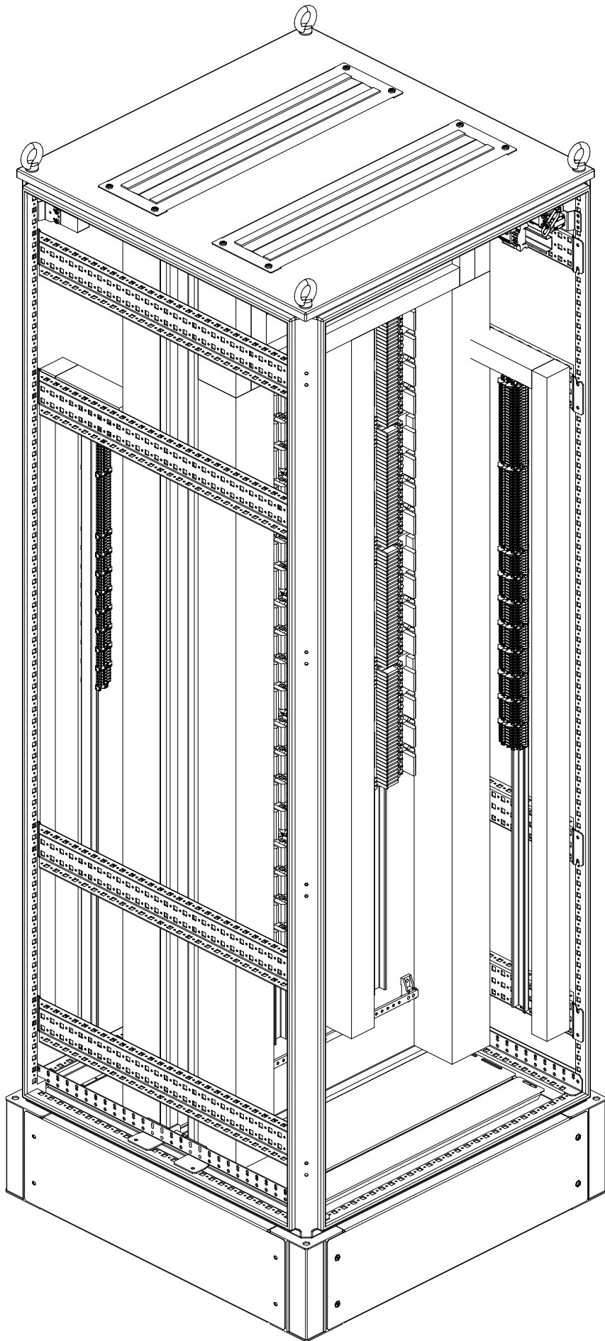
СВ изометрия
