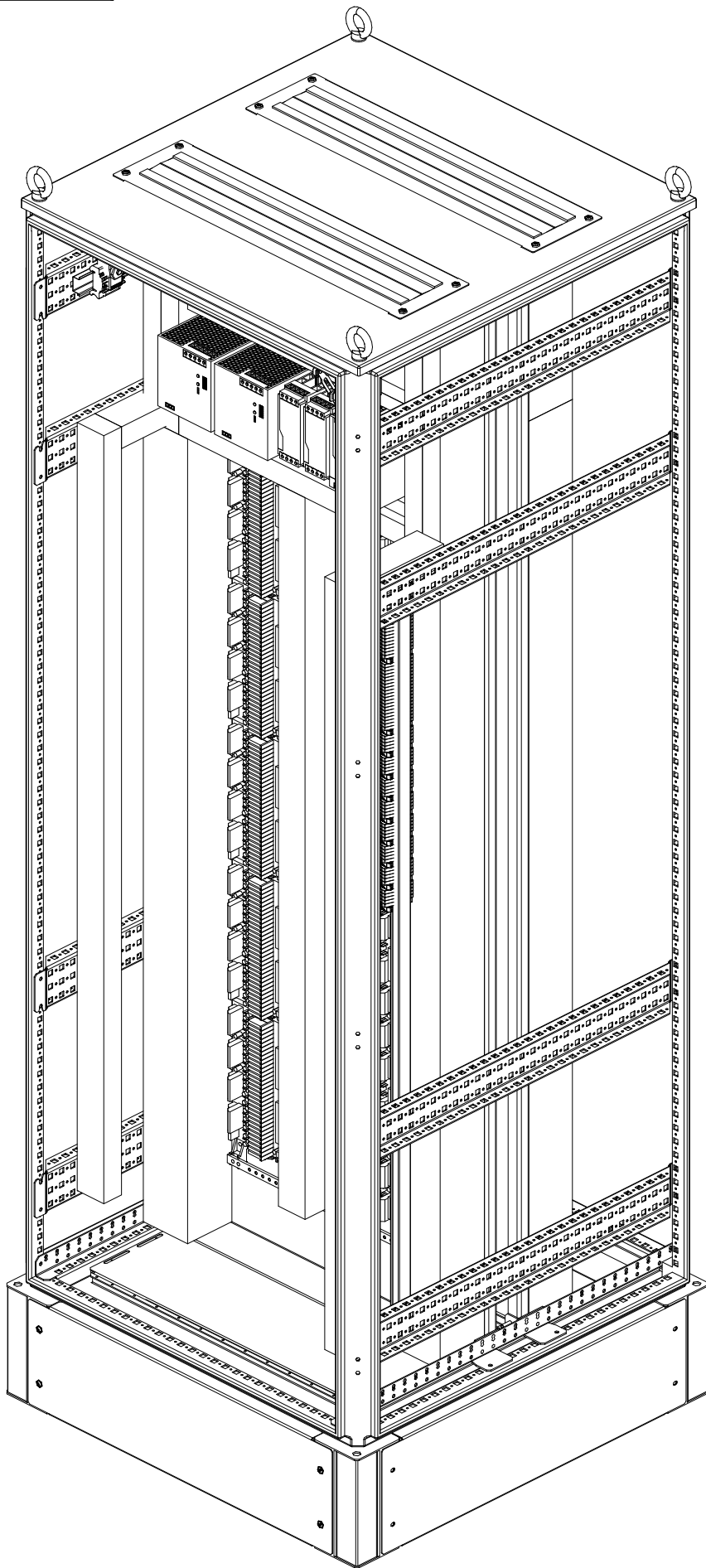
ЮВ изометрия
